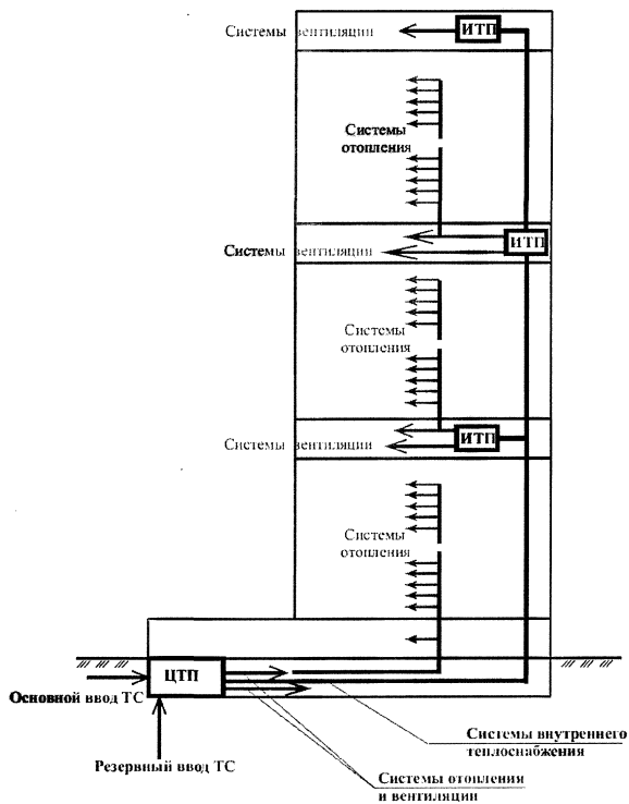
Рисунок 5.1 – Схема теплоснабжения высотного здания от централизованного источника
